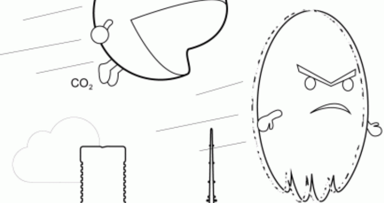
VOC
