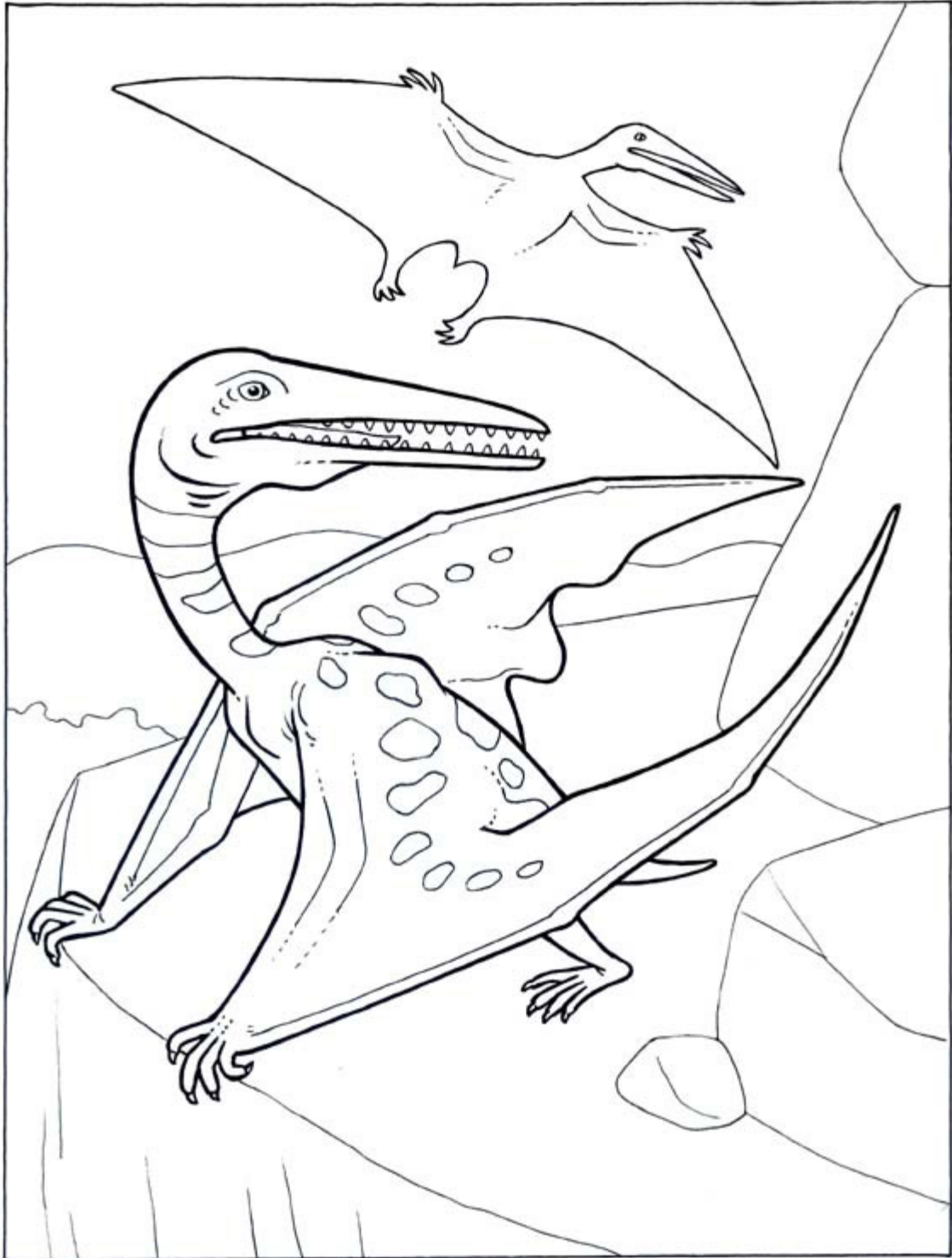
Pteradactyl, a flying dinosaur, Jurassic
