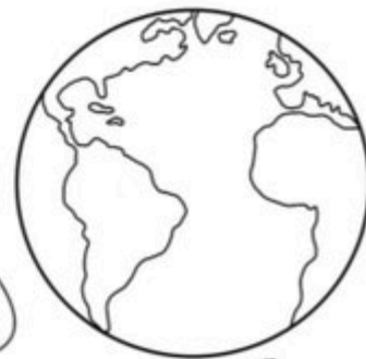
earth
