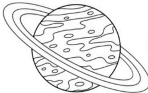
uranus
